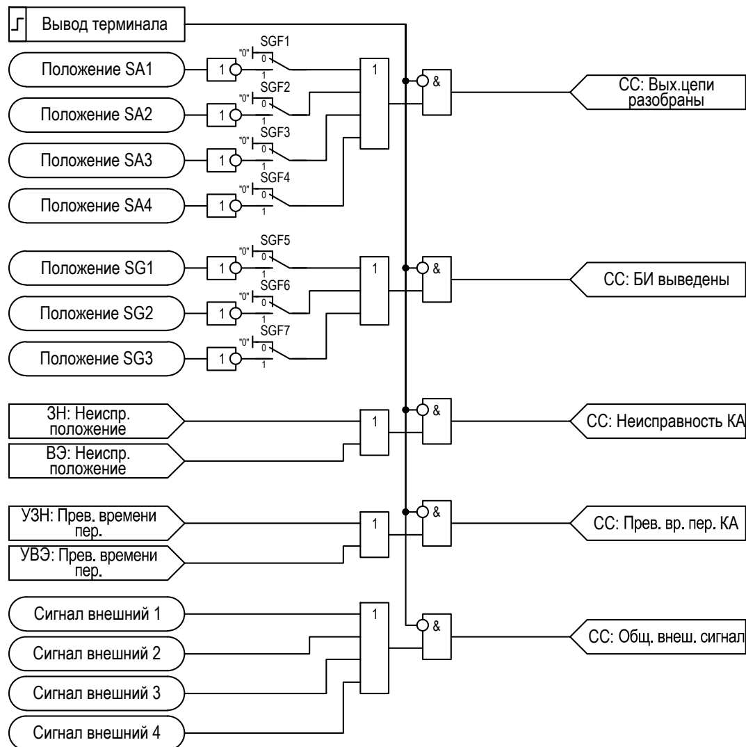
Рисунок 2.35 – Функциональная схема «CC»
