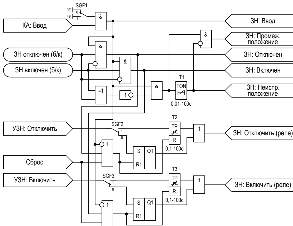
Рисунок 2.26 – Функциональная схема «ЗН»
